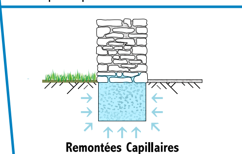
Cas de figure classic, traitement des remontées capillaires par l'intérieur ou l'extérieur
