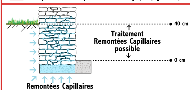
Attention si la différence entre le niveau du sol intérieur et extérieur est supérieur à 40 cm : procéder à un cuvelage (voir page 16-17)
